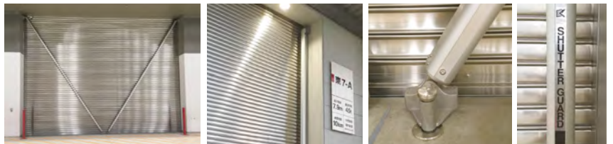
東京ビッグサイト②新東7・8展示棟 V型 シャッターサイズ:W9,830×H8,000(特殊対応品)
